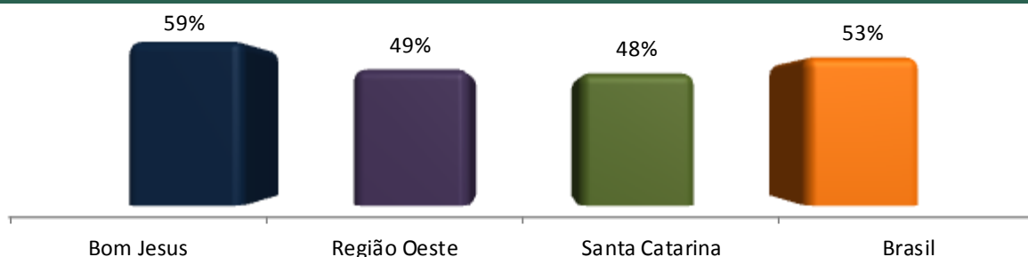
Gráfico 34 - Taxa de crescimento acumulada da frota de veículos, segundo Bom Jesus, Região Oeste, Santa Catarina e Brasil, no período de 2007 a 2012
